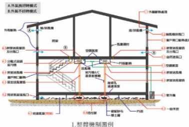
圖 33 AGS1 構造示意
