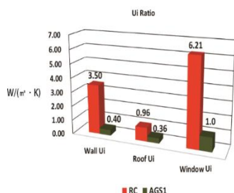
圖 30 AGS1 與 RC 構件之 U_i 對照表
