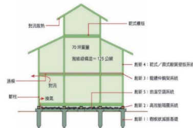
圖 23 雅緻創新結構系統示意圖
