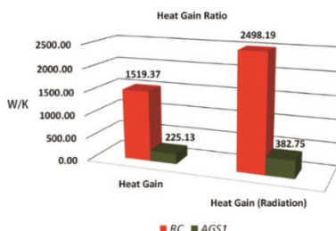
圖 31 AGS1 與 RC 熱得對照表
