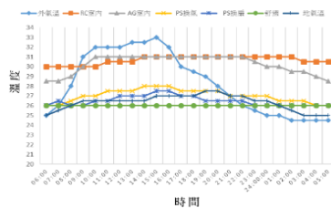
圖 40 AGS1 夏季溫度量測
