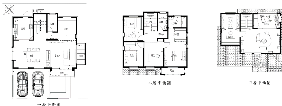
圖 8 各層平面圖
