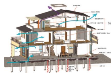
圖 24 雅緻創新複合構造示意圖
